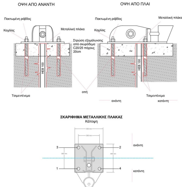
Εικόνα 6: Περιοχή IV - Λεπτομέρεια θεμελίωσης
