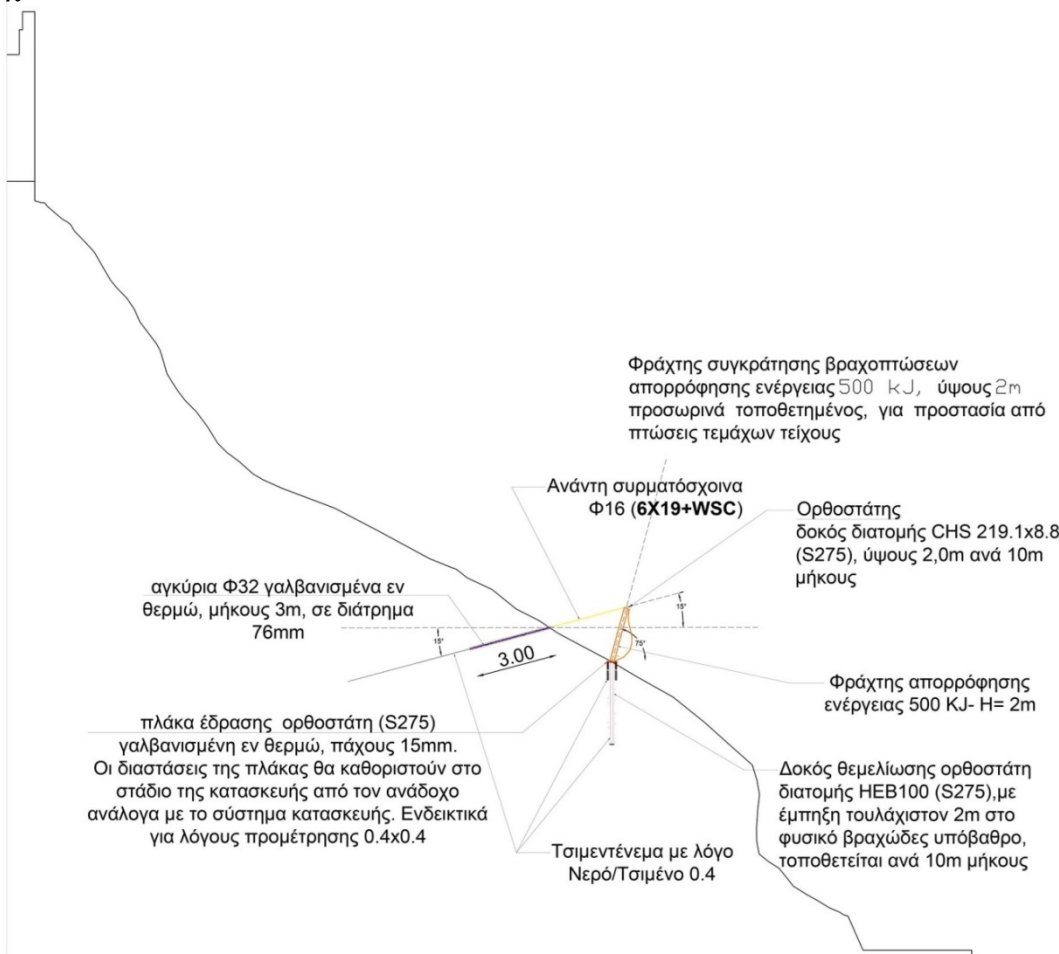
Εικόνα 2: Περιοχή IV - Διατομή
