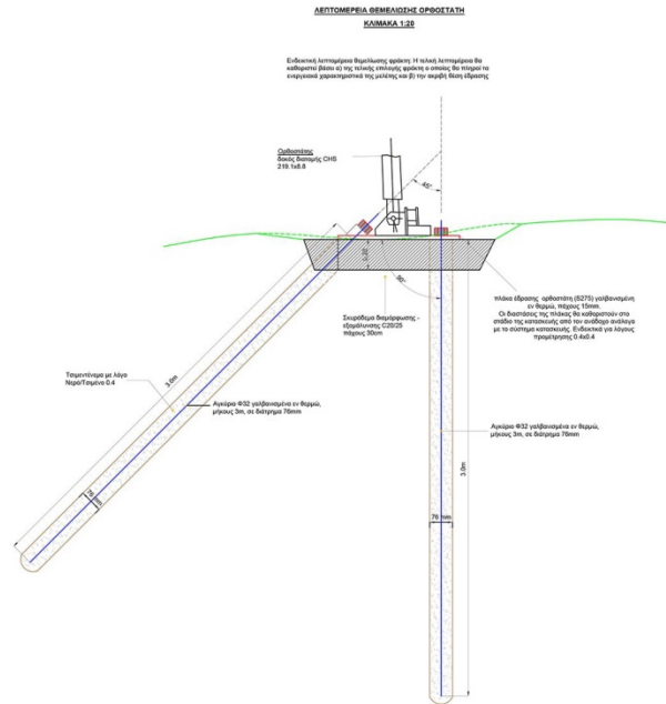
Εικόνα 4: Περιοχή VI - Λεπτομέρεια θεμελίωσης
