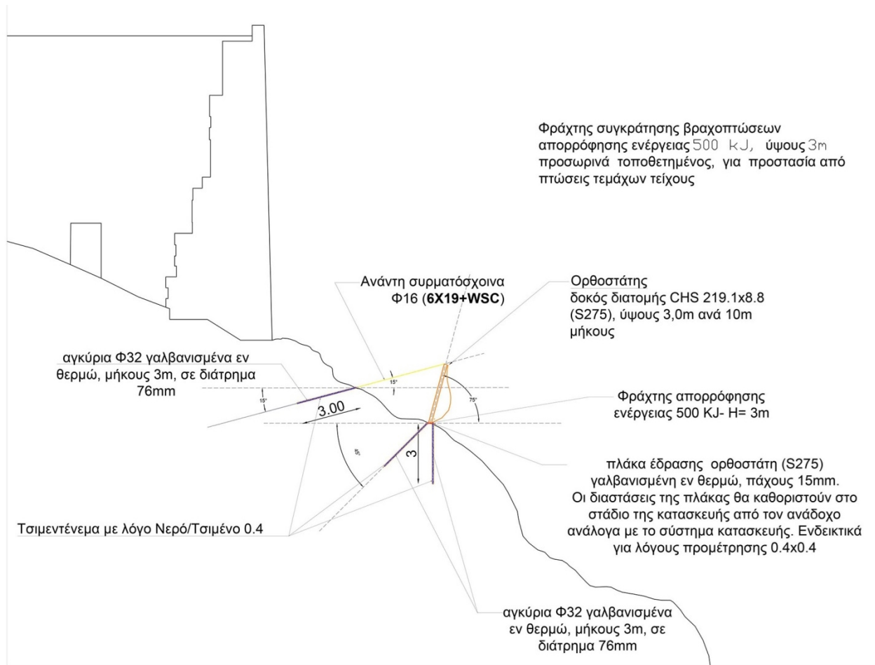
Εικόνα 3: Περιοχή VI - Διατομή
